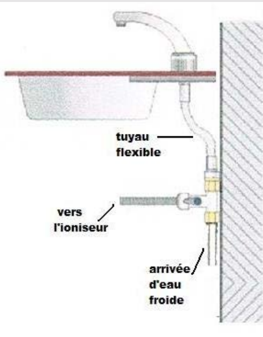
Shéma d'emplacement
